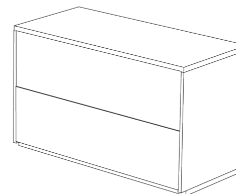
cod.STR ACC 014.1 CASSETTIERA 2 CASSETTI L800 P400 H480
